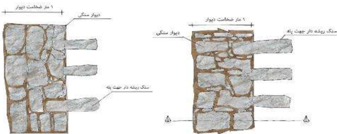
تصویر ۱۴. جزئیات ساخت پله برای دسترسی به تلان‌ها (ماخذ: نگارنده)
